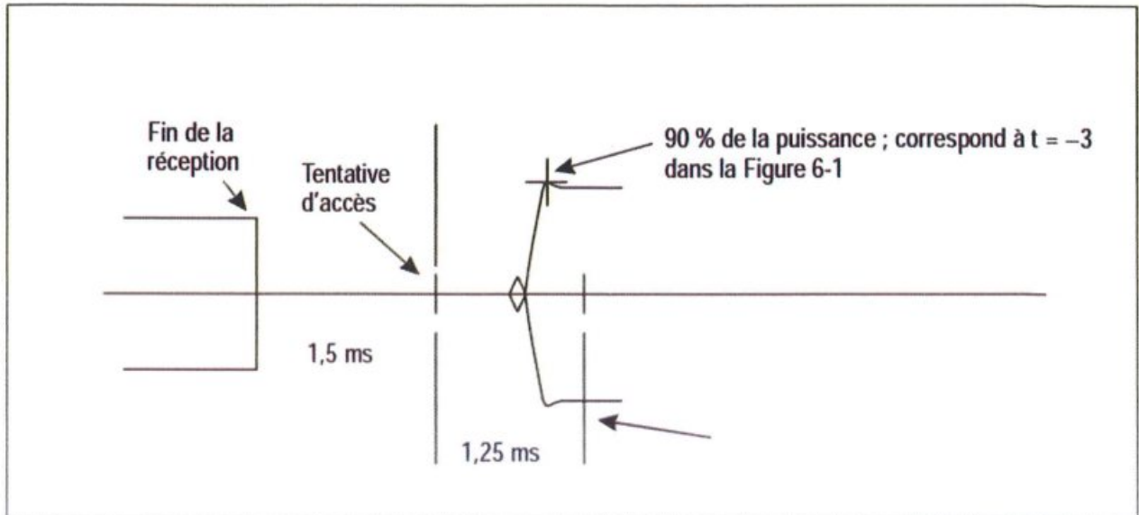
Figure 6-3. Temps de retournement réception-émission
