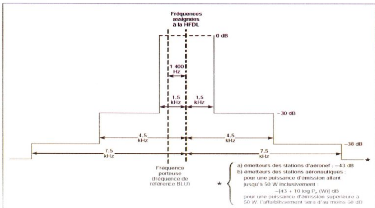
Figure 11-1. Limites spectrales requises (puissance de crête) pour les émetteurs des stations d'aéronef et des stations sol HF/DL.
