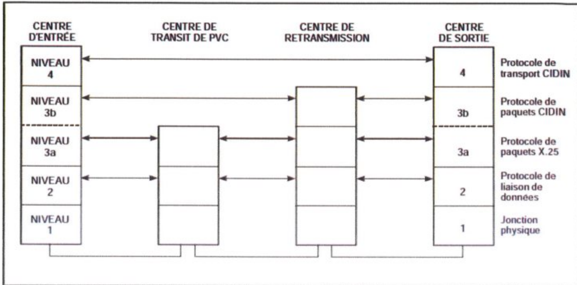
Figure 8-1. Niveaux de protocole CIDIN
